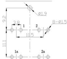
印制板开孔尺寸(±0.1mm)
